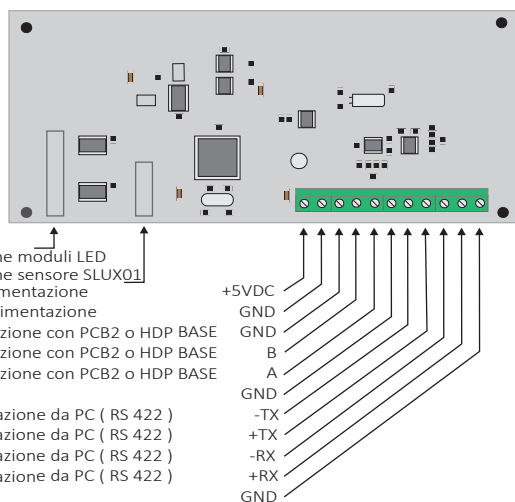
Scheda di controllo GRGB, connessioni
