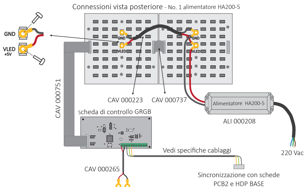
Collocazione scheda GRGB
